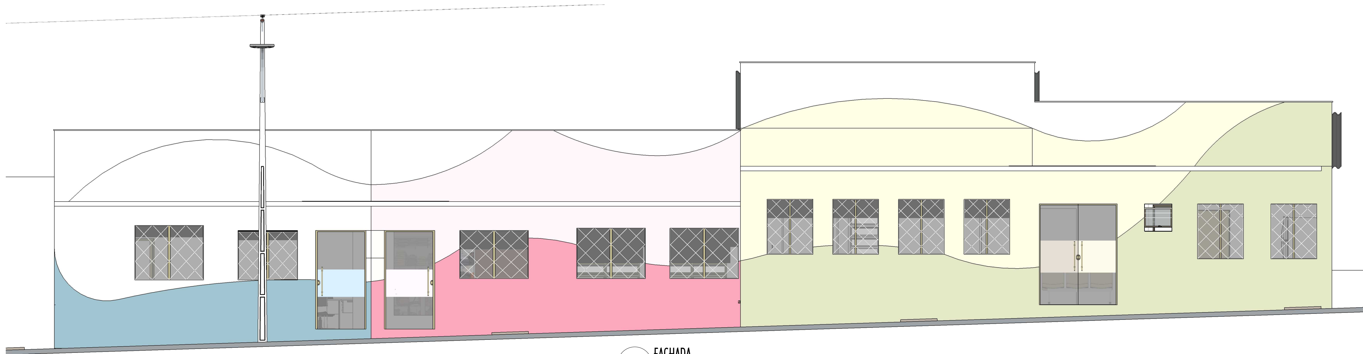
11 FACHADA Escala 1:50
